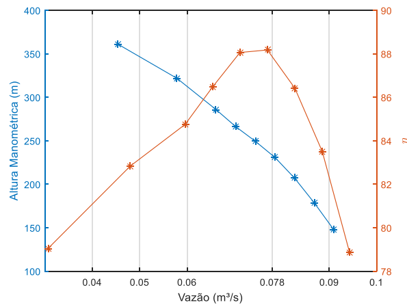
Figura 2 – Curvas de altura manométrica e rendimento como função da vazão volumétrica. a) 1250 rpm. b) 1500 rpm. c) 2000 rpm
