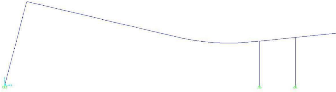
Figura 17. Corte do conjunto formado pelo pilar frontal, viga central e paredes estruturais. Desenho do autor. Programa SAP 2000.
