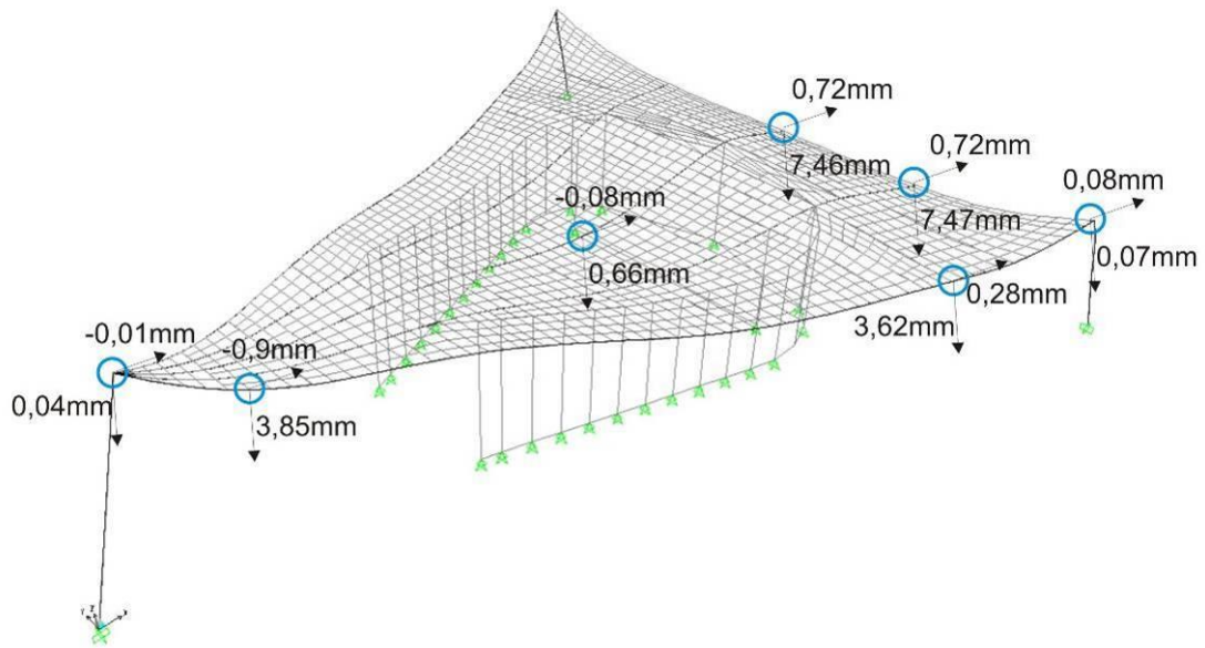
Figura 28: Diagrama de Deformações. Desenho do autor. Programa SAP 2000.
