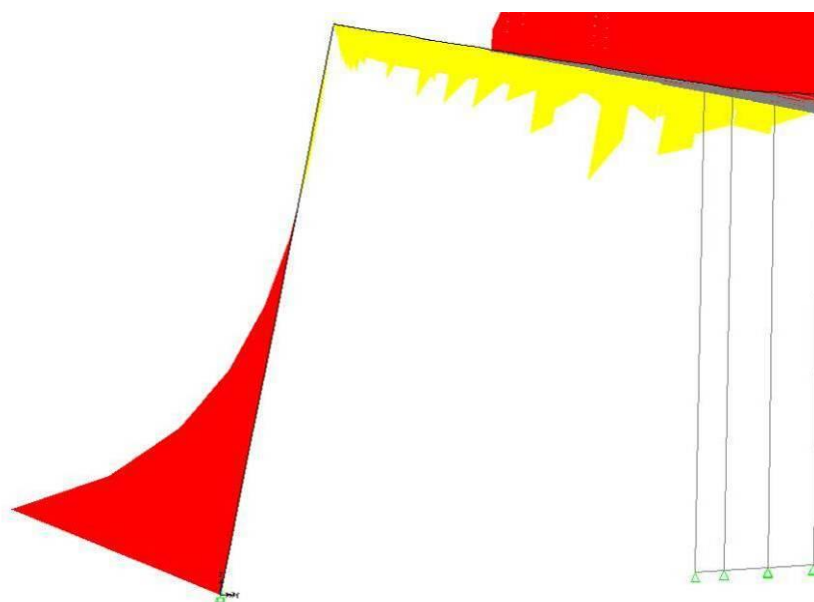
Figura 24. Diagrama de Momentos Fletores – detalhe do Pilar Frontal. Desenho do autor. Programa SAP 2000.
