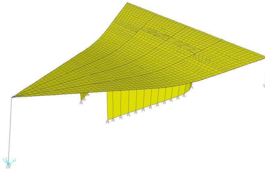
Figura 21. Sistema Estrutural da Igrejinha Nossa Senhora de Fátima. Desenho do autor. Programa SAP 2000.
