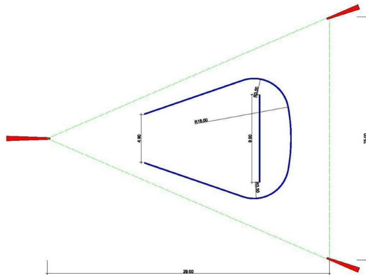
Figura 2. Planta da Igreja Nossa Senhora de Fátima. Desenho do Autor – adaptado de planta original cedida pelo IPHAN-DF.
