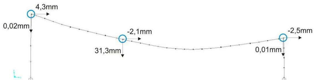
Figura 16. Diagrama de Deformações. Desenho do autor. Programa SAP 2000.
