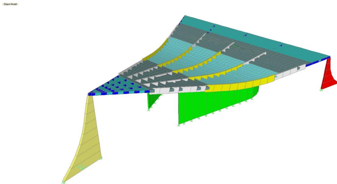
Figura 12. Perspectiva esquemática da estrutura da Igreja. Desenho do autor. Programa SAP 2000.
