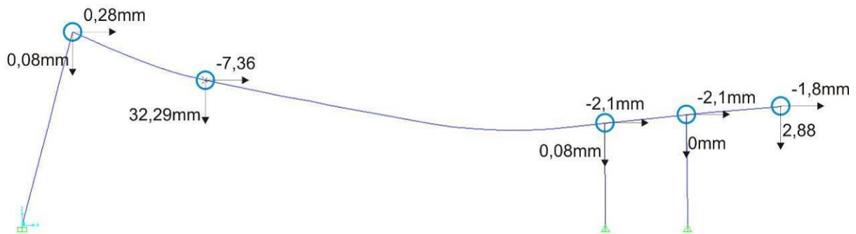
Figura 20. Diagrama de Deformações do conjunto formado pelo pilar frontal, viga central e paredes estruturais. Desenho do autor. Programa SAP 2000.
