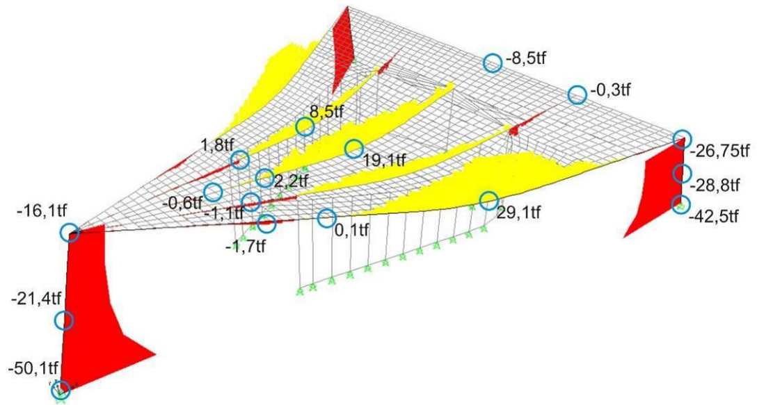
Figura 22. Diagrama de Forças Normais. Desenho do autor. Programa SAP 2000.
