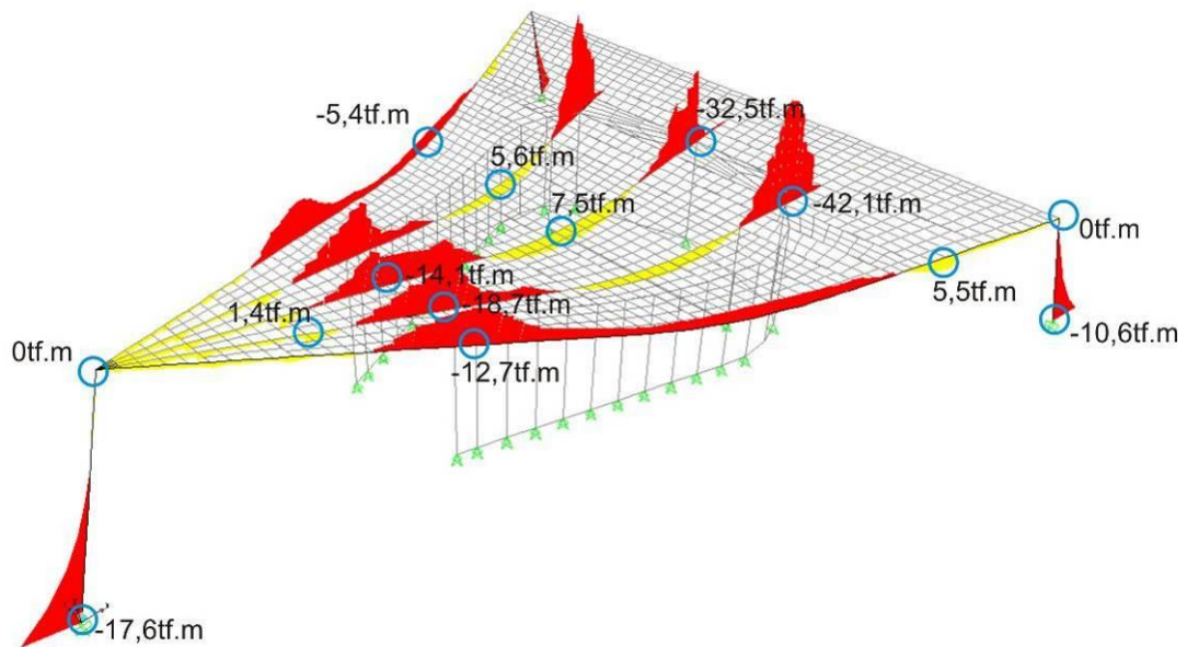
Figura 23. Diagrama de Momentos Fletores. Desenho do autor. Programa SAP 2000.
