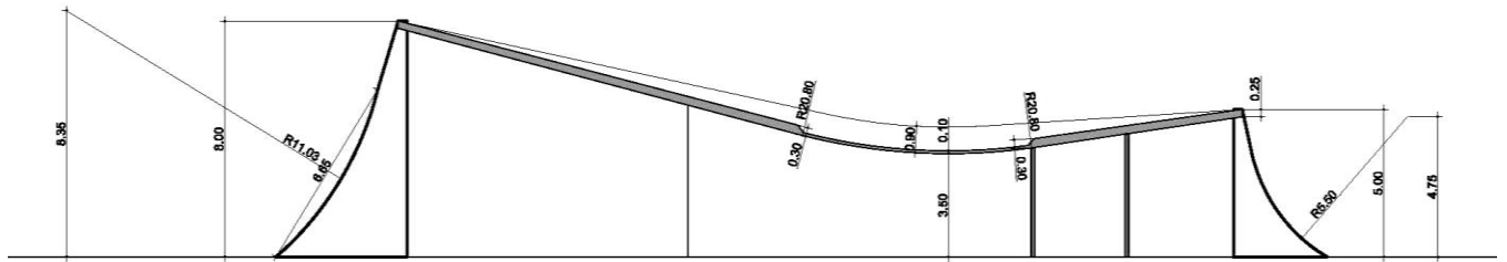
Figura 7. Corte Longitudinal da Igrejinha Nossa Senhora de Fátima. Desenho do autor – adaptado de planta original (IPHAN).
