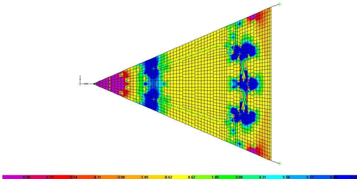
Figura 27. Diagrama de Momentos Fletores na direção “y” na laje da Igreja Nossa Senhora de Fátima. Desenho do autor. Programa SAP 2000.
