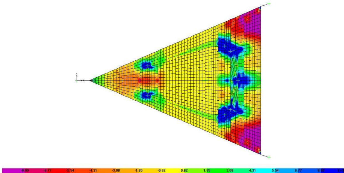
Figura 26. Diagrama de Momentos Fletores na direção “x” na laje da Igreja Nossa Senhora de Fátima. Desenho do autor. Programa SAP 2000.
