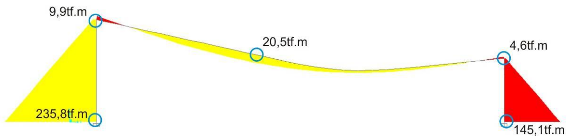
Figura 15. Diagrama de Momentos Fletores. Desenho do autor. Programa SAP 2000.
