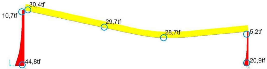
Figura 14. Diagrama de Forças Normais. Desenho do autor. Programa SAP 2000.
