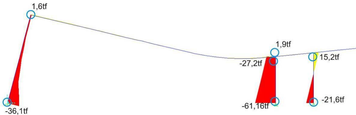
Figura 18. Diagrama de Forças Normais do conjunto formado pelo pilar frontal, viga central e paredes estruturais. Desenho do autor. Programa SAP 2000.
