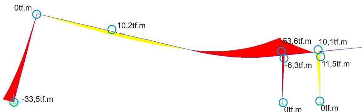
Figura 19. Diagrama de Momentos Fletores do conjunto formado pelo pilar frontal, viga central e paredes estruturais. Desenho do autor. Programa SAP 2000.
