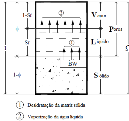
Figura 1. Repartição volumétrica das fases do concreto
