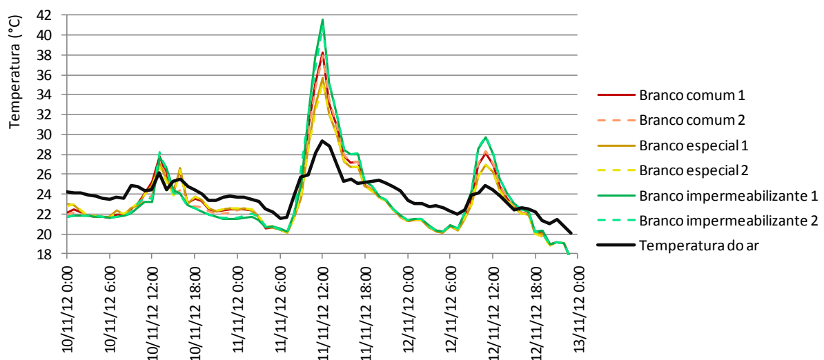
Figura 8: Temperatura superficial das amostras brancas e temperatura do ar.
