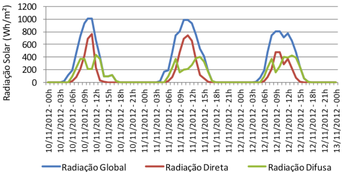
Figura 6: Radiação solar global obtida nos piranômetros do Lepten.
