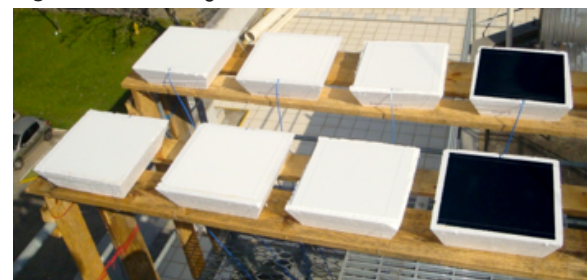
Figura 3: Plataforma posicionada na cobertura de prédio da UFSC.
