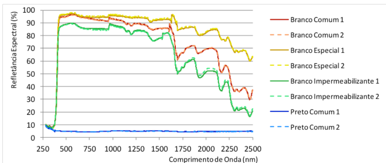
Figura 4: Refletância espectral das amostras.
