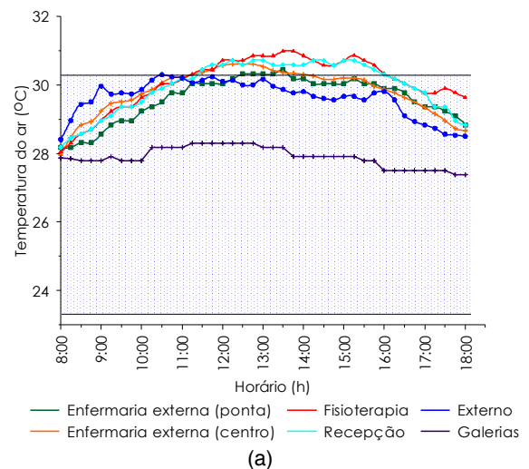
Gráfico 1: Temperatura do ar média (°C) externa e nos ambientes internos e limites superior e inferior recomendado pela ASHRAE (a) ambientes orientados para nordeste e (b) sudoeste no Sarah de Salvador
