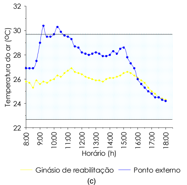
Gráfico 2: Temperatura do ar (°C) externa e nos ambientes internos para o dia 13/07/2010 e limites superior e inferior recomendado pela ASHRAE (a) ambientes para leste, (b) oeste e (c) sul no Sarah do Rio de Janeiro.
