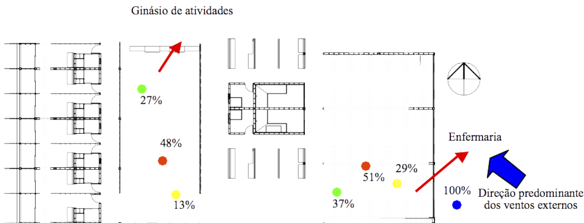
Figura 12: Velocidade do ar no interior em função do vento externo no Sarah - Rio
