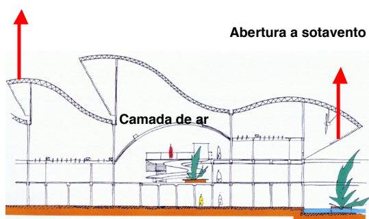
Figura 10: Corte do hospital do Rio
