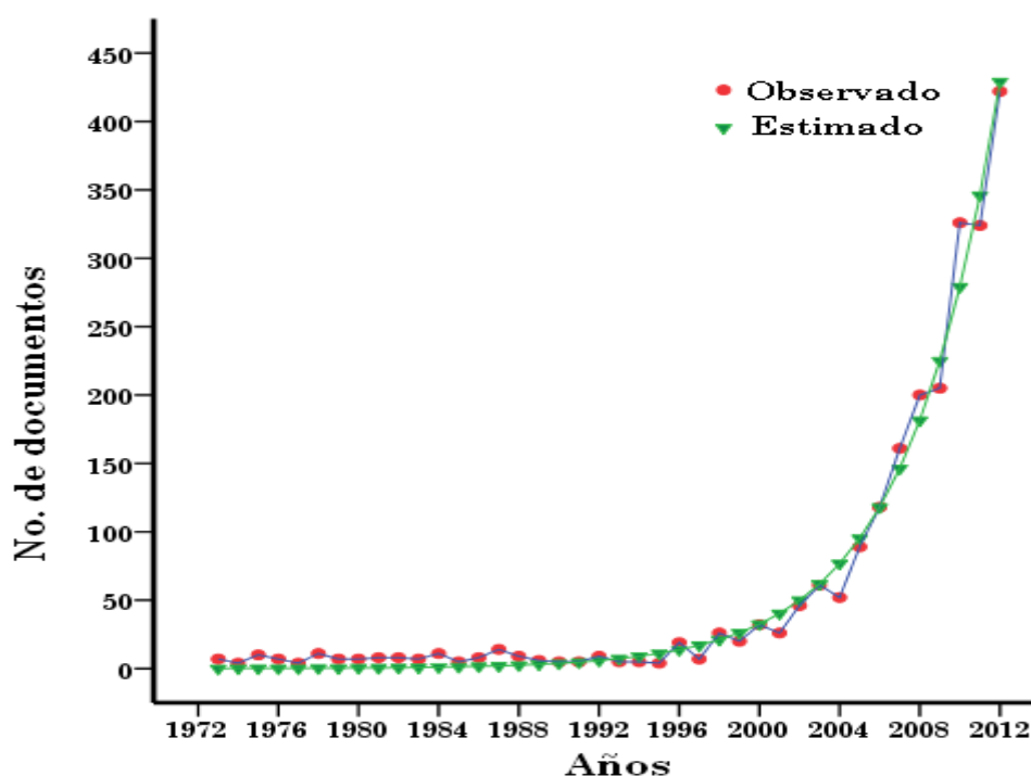
Figura 3. Gráfico de los valores observados y estimados.
